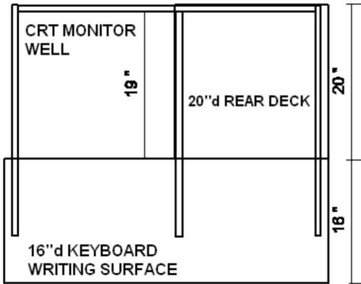
TOP
